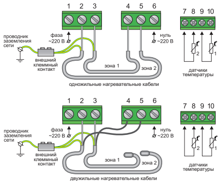
Рис. 8 Схема подключения к трехпроводной электрической сети
