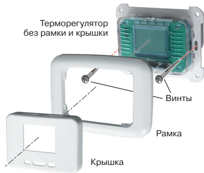
Рис. 10 Установка терморегулятора
