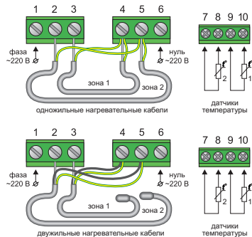
Рис. 7 Схема подключения к двухпроводной электрической сети
